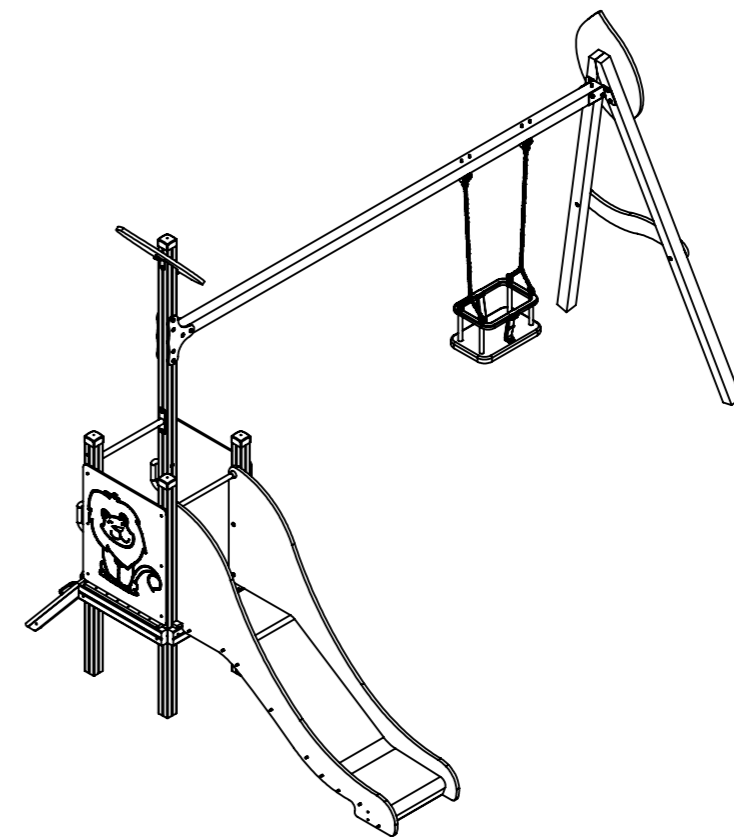
CASA DE JUEGOS MODELO DENIA REF 239D - DIMENSIONES GENERALES
