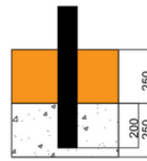
Suelo blando (tierra, arena) de 250mm Dado de hormigón de 450x450x250mm
