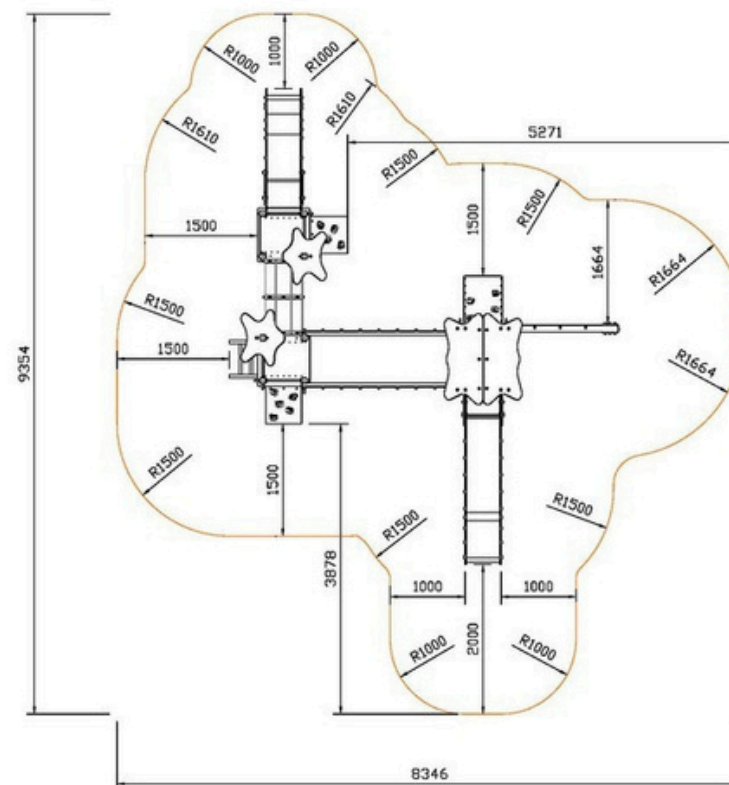
CASA MODELO FLORENCIA REF. 2210 ÁREA DE SEGURIDAD
