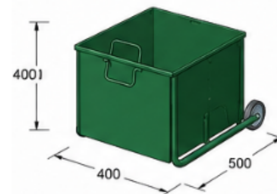
DETALLE CAJA CONTRAPESO
