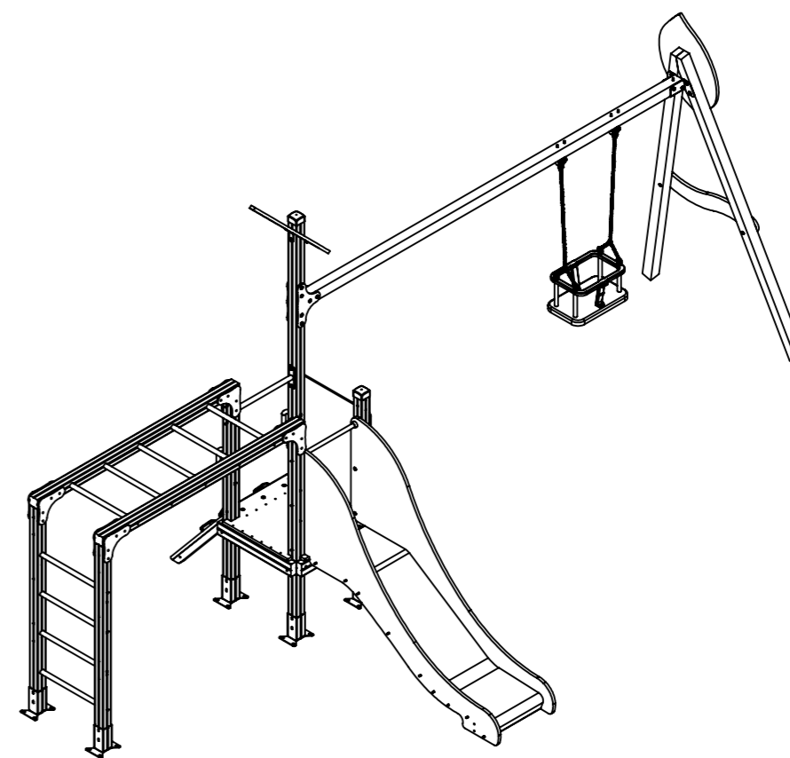
CASA DE JUEGOS MODELO ESTEPONA REF 239E - DIMENSIONES GENERALES
