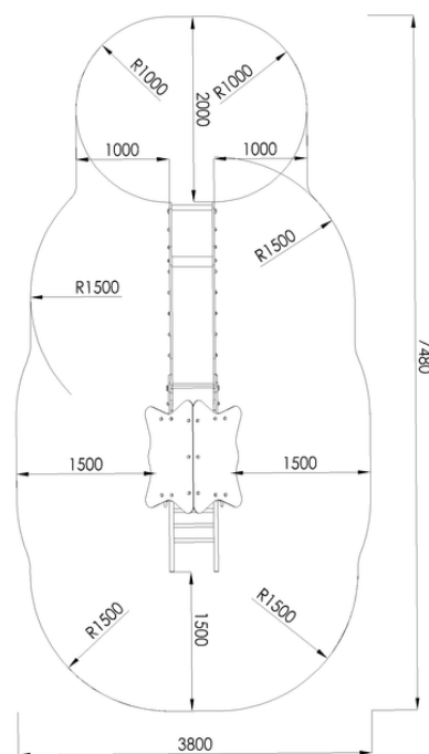
CASA DE JUEGOS MODELO SORIA REF. 296-D ÁREA DE SEGURIDAD
