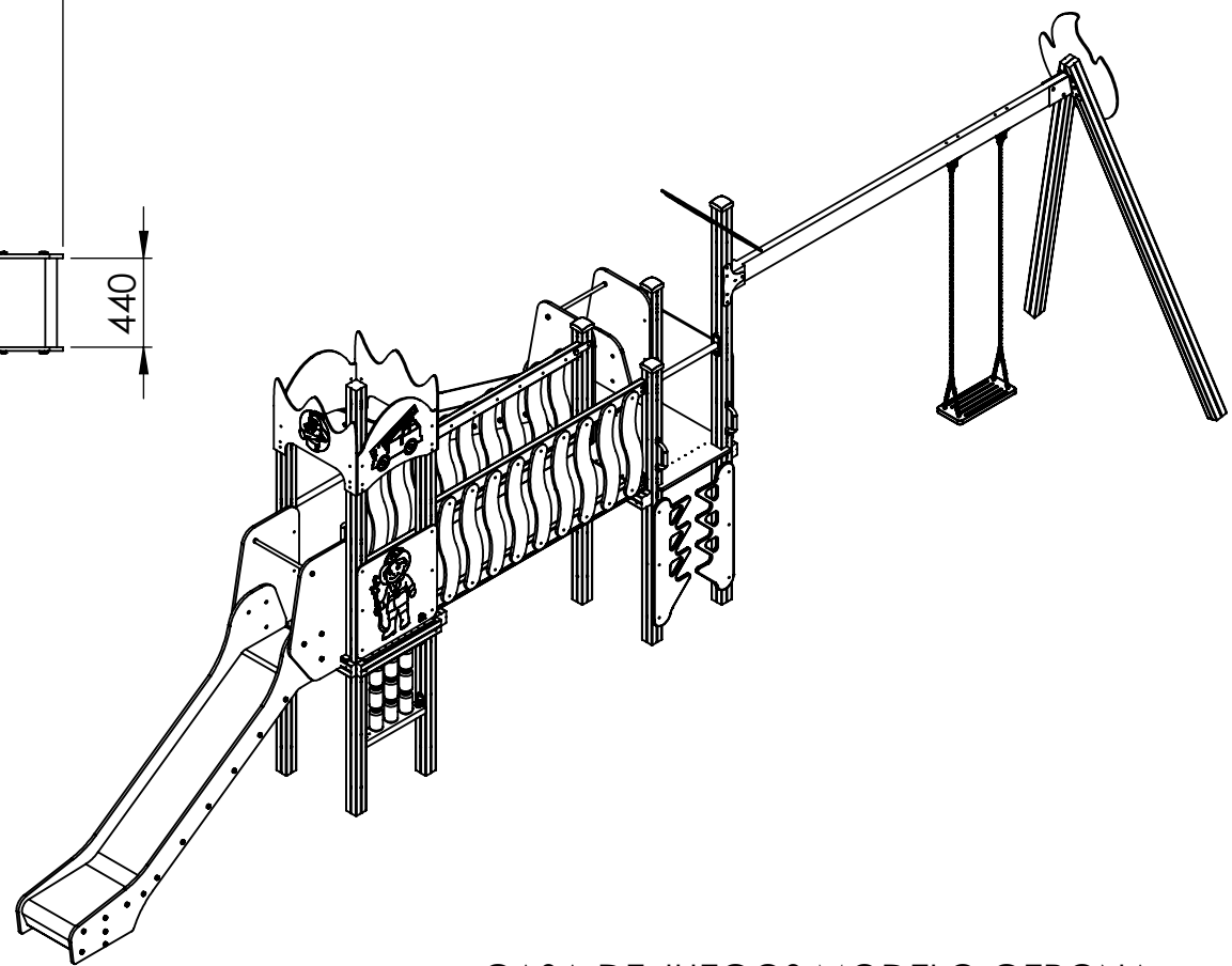
CASA DE JUEGOS MODELO GERONA REF 292G - DIMENSIONES GENERALES
