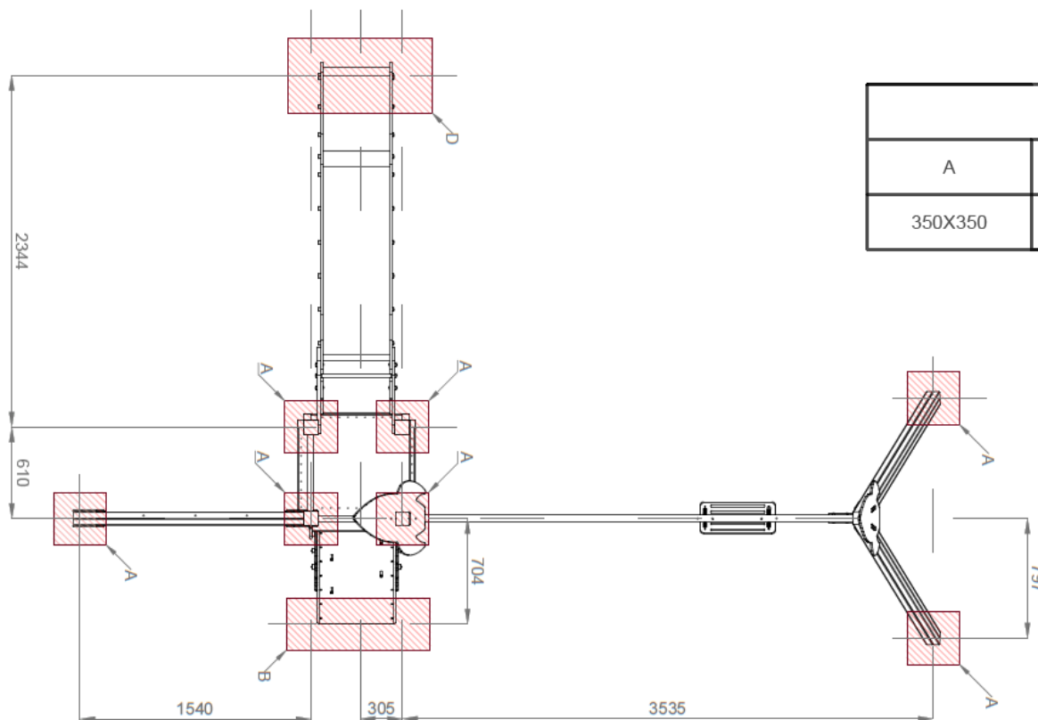
Cotas Cubos Cimentación (mm)
