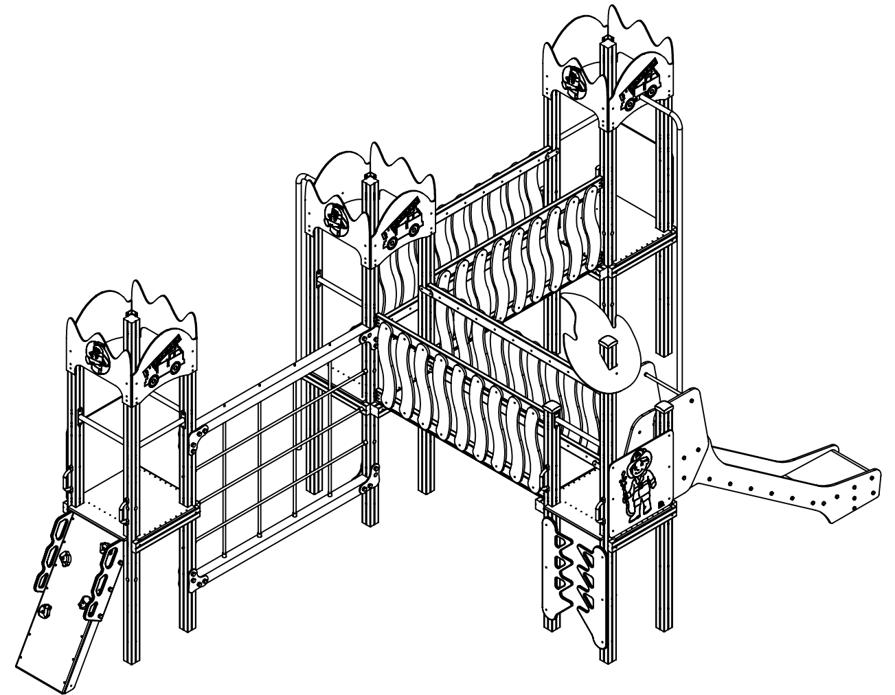
CASA DE JUEGOS MODELO SEGOVIA REF. 292B - DIMENSIONES GENERALES
