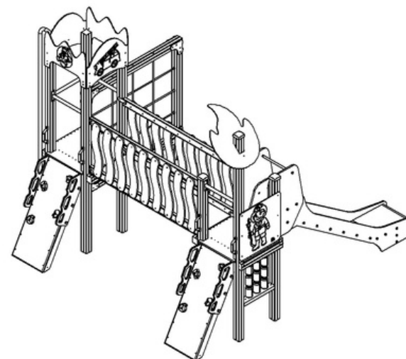
CASA DE JUEGOS MODELO VALLADOLID REF 291A - DIMENSIONES GENERALES
