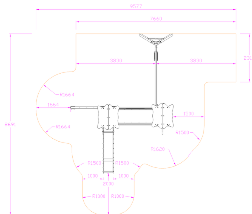
CASA DE JUEGOS MODELO FORMENTERA REF. 292-F ÁREA DE SEGURIDAD
